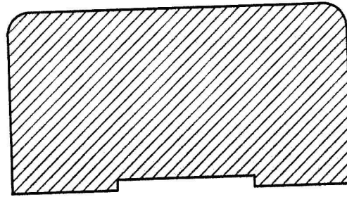
DE 75 38 x 70 mm N : RM8.00
