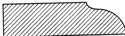
SK 78-70 70x22 mm N : RM3.15 K, KSK : RM3.15
