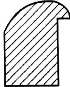
DE 0146 24 x 20 mm N: RM 1.15 K, KSK: RM 1.15
