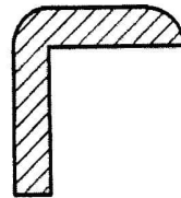
DE 2221 24 x 23 mm N: RM1.35 KSK: RM1.35
