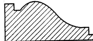
DE 1845 18 x 45 mm N : RM 2.30 K, KSK : RM 2.30
