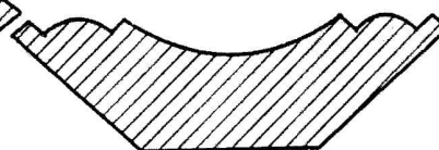
DE 1158 58x21 mm N : RM 2.75 K, KSK : RM2.75
